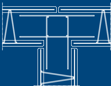
Aansluiting dwarswand
