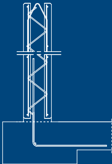
Vloeraansluiting
