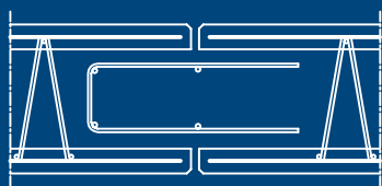
Voegdetail
