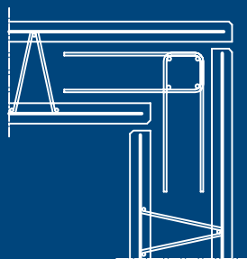
Hoekaansluiting
