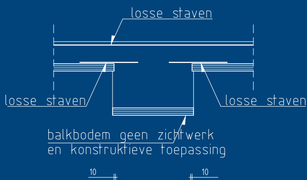
Aansluitdetail breedplaatvloer-balkbodem*
