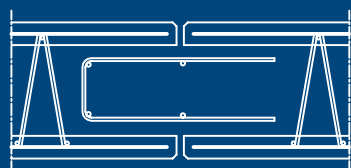
Voegdetail
