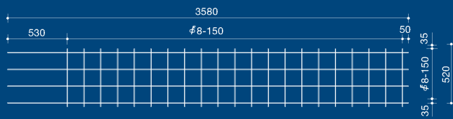
Wapeningsmat voor funderingsstrook van 600 mm breed
